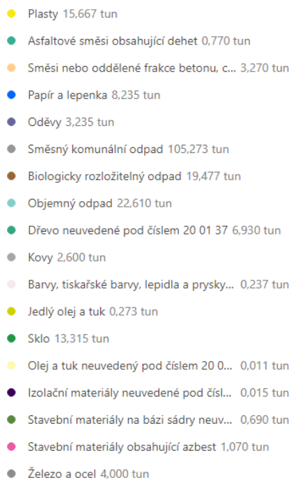
Sumarizační graf
